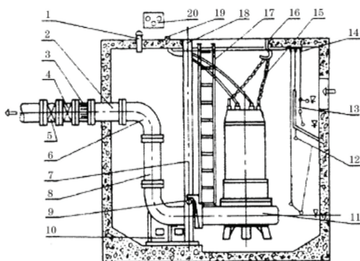
Рис. 8 Стационарная установка
